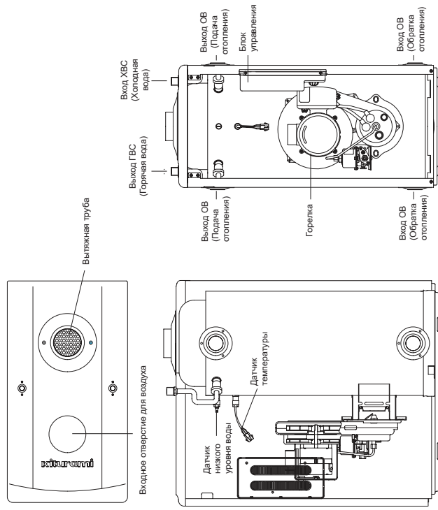
■ Схема внешнего вида продукта STS-13R/17R/21R (Жидкотопливный)
